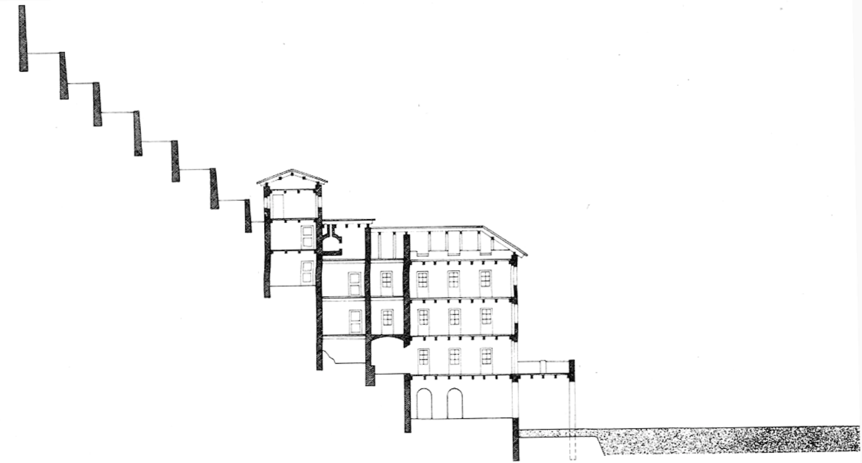
Sezione B-B
